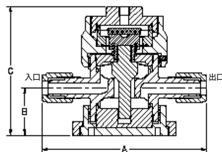
UPBM 1/2" 空気式
