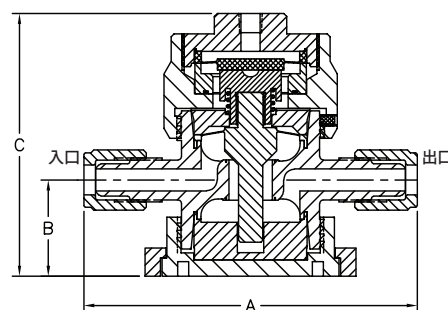
UPBM 1/2" 空気式
